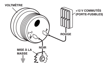
Figure 4. Raccordement du voltmètre
