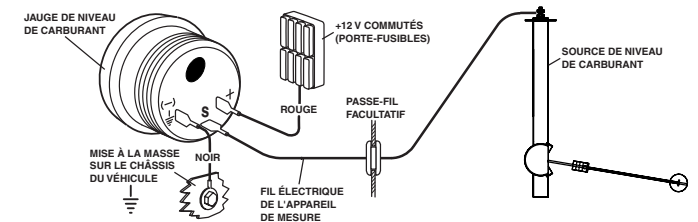
Figure 6. Raccordements de la jauge de niveau de carburant
